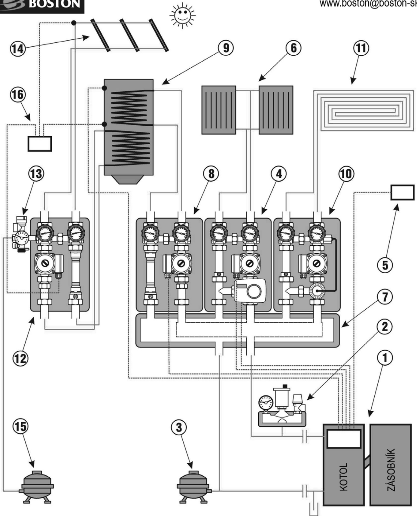
Doporučené zapojenie kotla do vykurovacieho okruhu pomocou hydraulických modulov s ohrevom TUV, podlahovým vykurovaním a solárnymi panelmi
